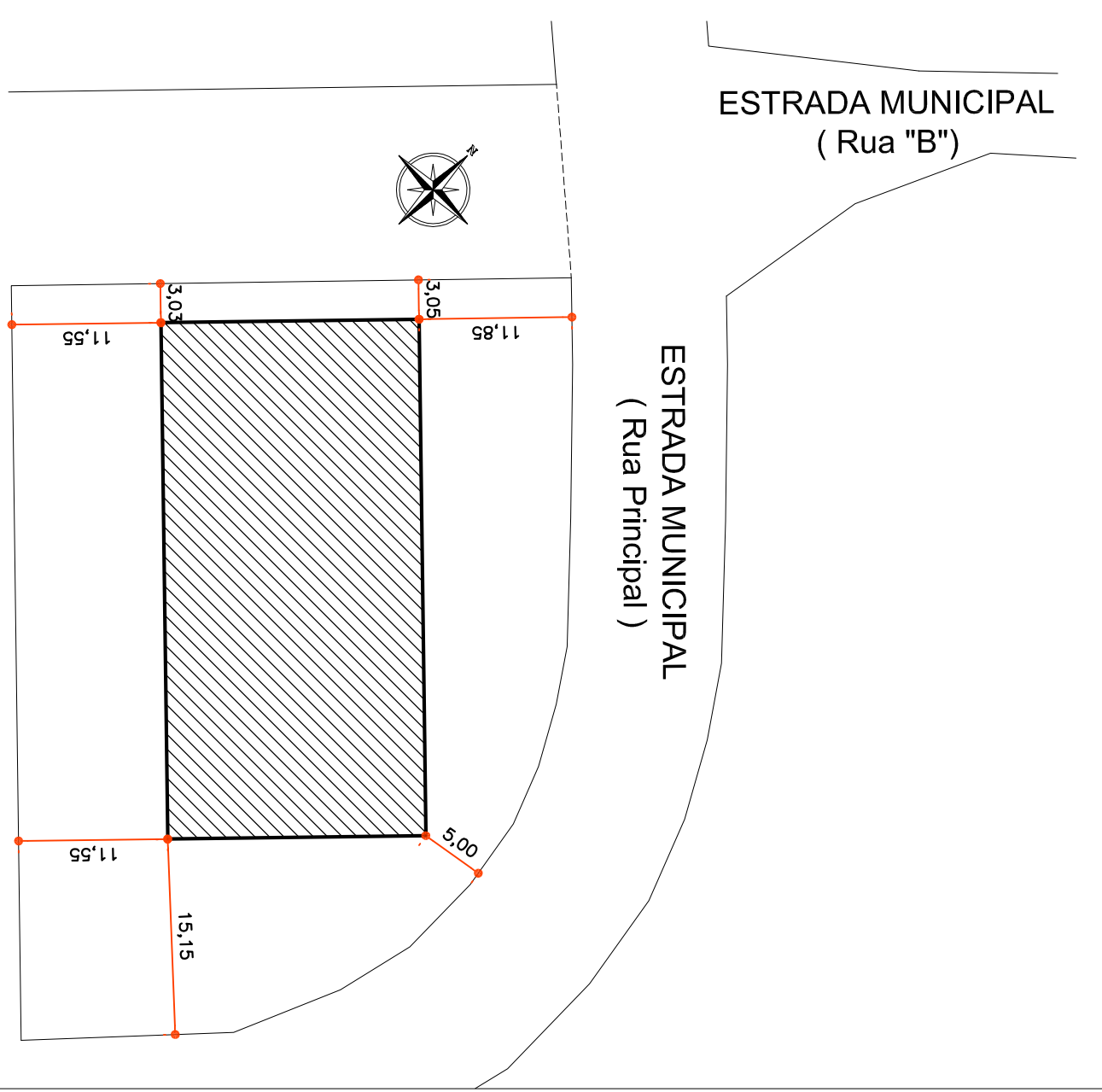
IMPLANTAÇÃO Esc.: 1/400
