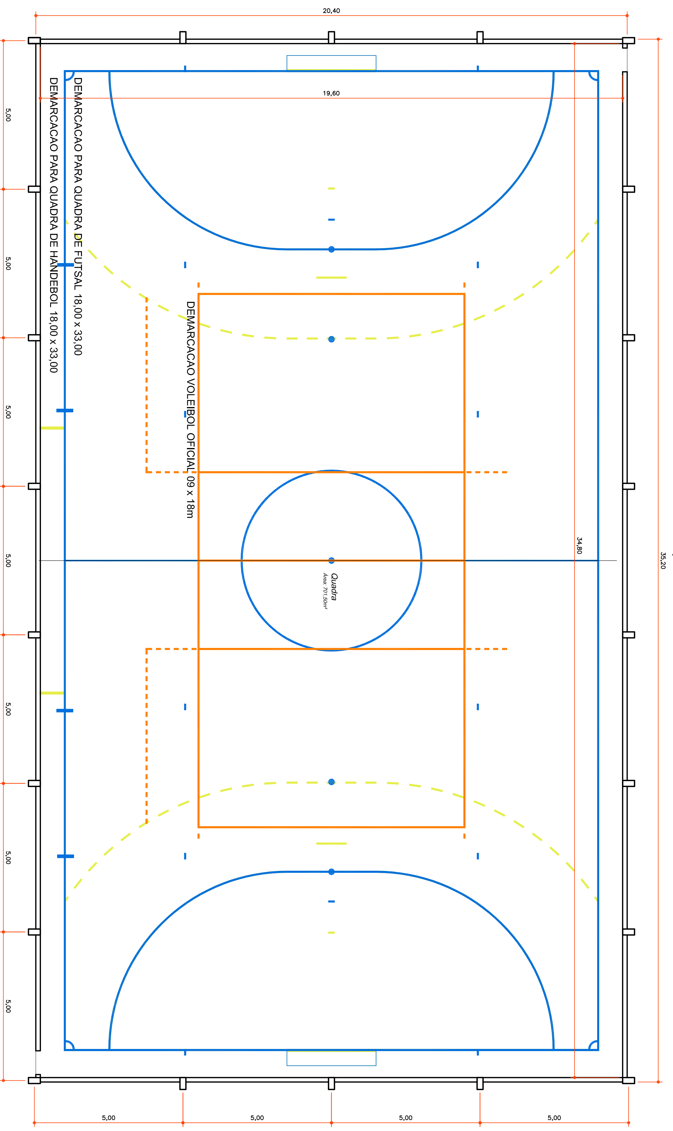
IMPLANTAÇÃO Esc.: 1/400
