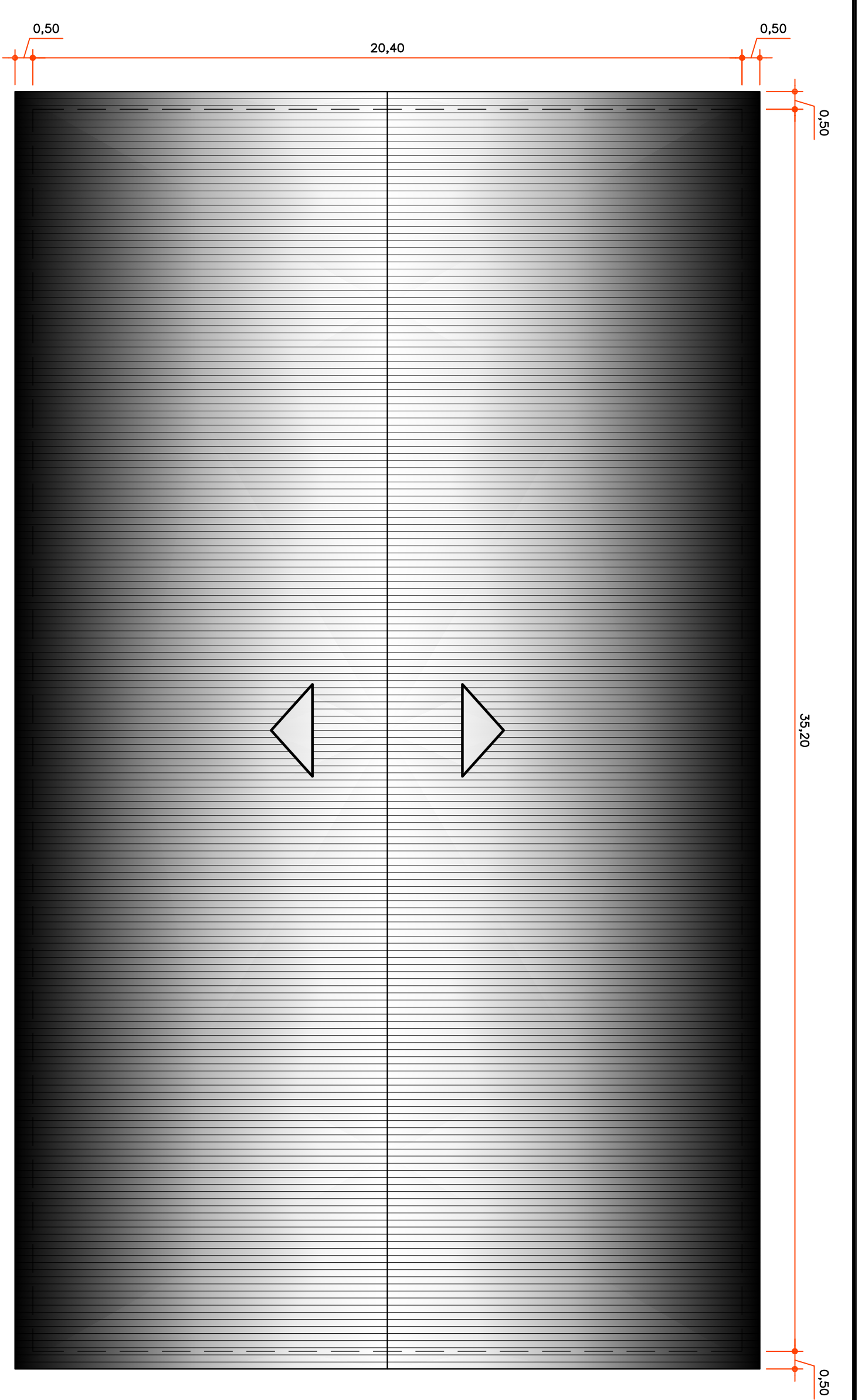
PLANTA DE COBERTURA Área: 774,68m² Esc.: 1/125
